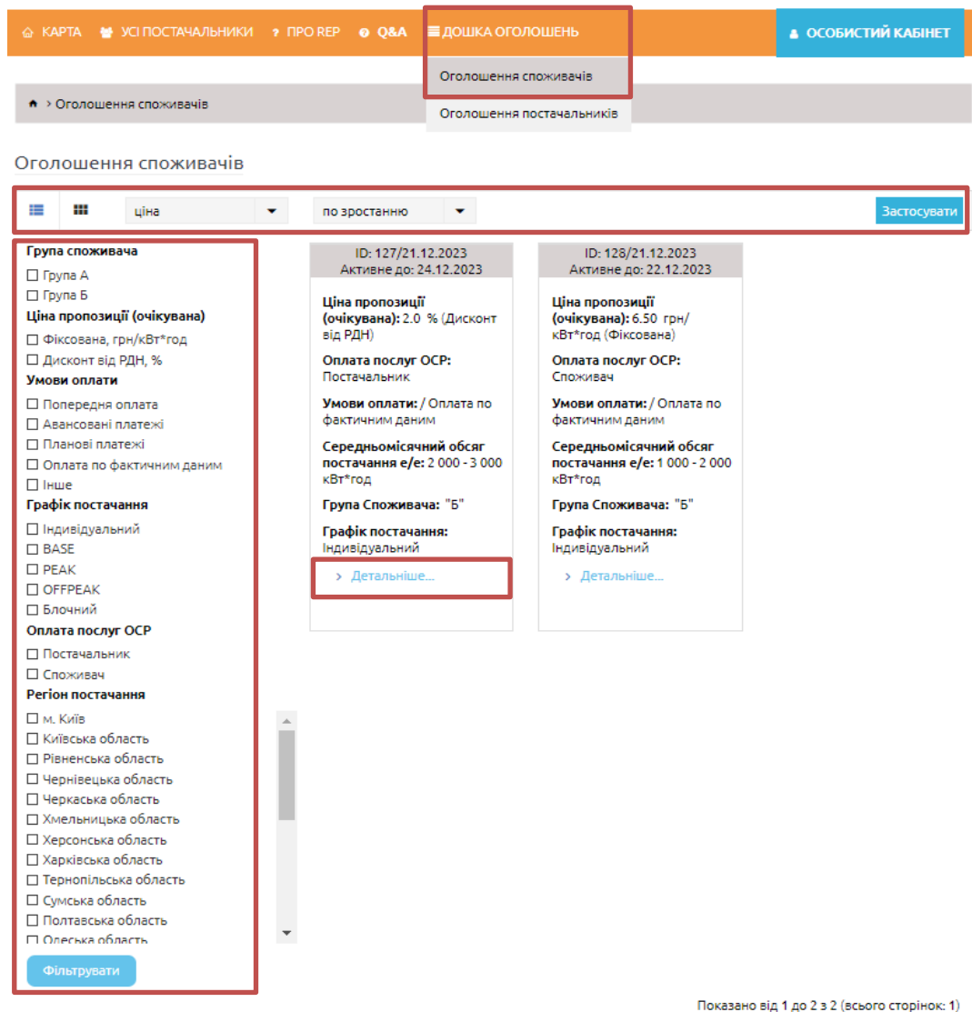
Рисунок 1.6 Інтерфейс розділу «Оголошення споживачів»
